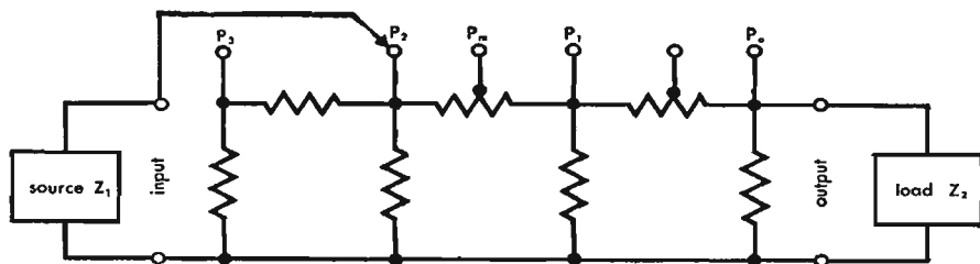
Fig. 15—Ladder attenuator.
