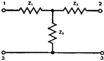
T or Y network
