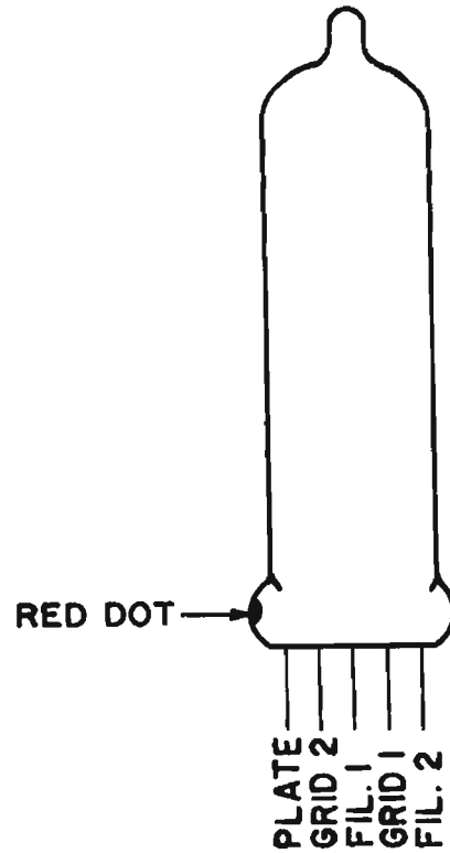
Fig. 20—Subminiature tube.
