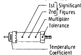
Fig. 33—Capacitor color code.
