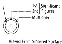
Fig. 33—Capacitor color code.
